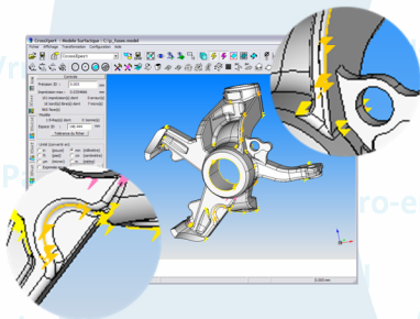
Défauts géométriques détectés par CrossXpert
